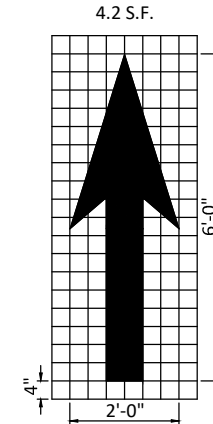
DETAIL 4 BIKE LANE ARROW N.T.S.
